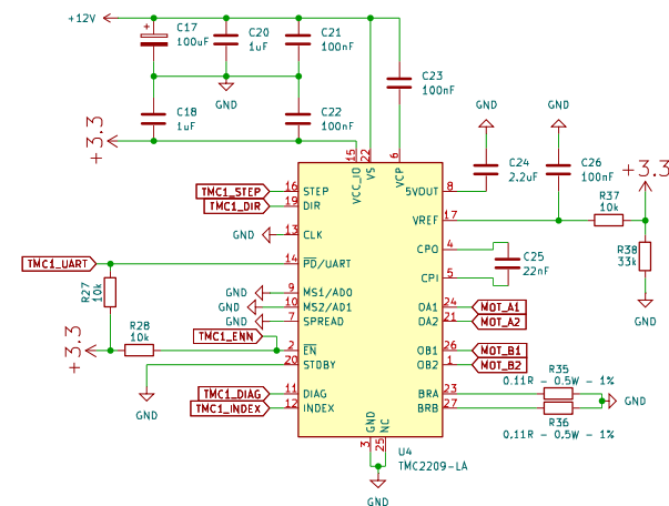
TMC 2209
